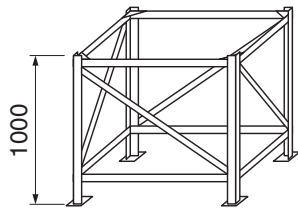
Podest PRC
