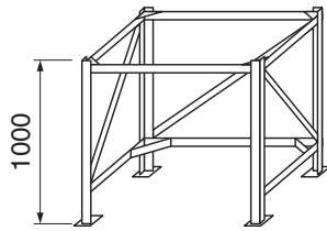
Podest PRA (einseitig offen)
