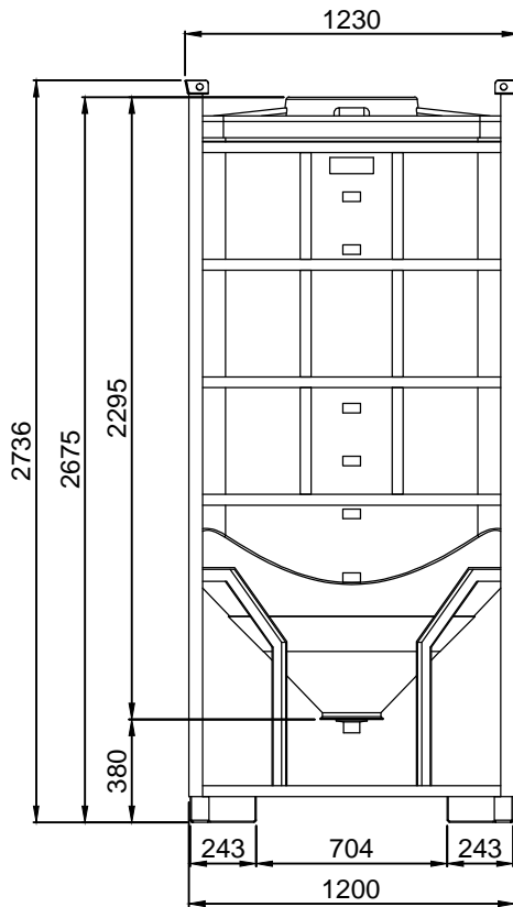
Innenbehälter
