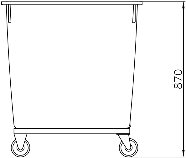
Fahrgestell
