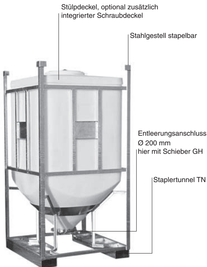
Container TB 21-2/P mit Staplertunnel TN + Schieber GH
