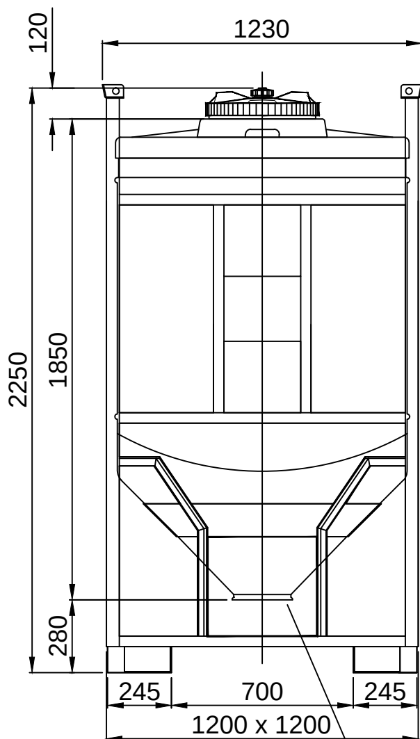
Innenbehälter
