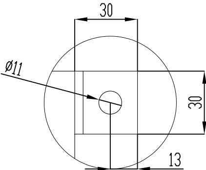
Detail F 1 : 2
